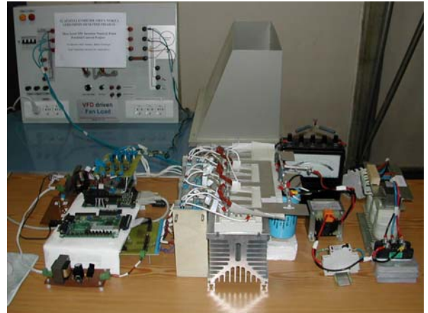
Şekil 9 Deneysel üç-düzeyle evirici sistemi ve havalandırıcı yük sistemi.
