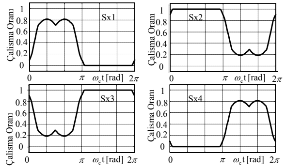
Şekil 5 Üç-düzeyle evirici yarı-iletken anahtarlarının çalışma oranları (x:U, V, W).
