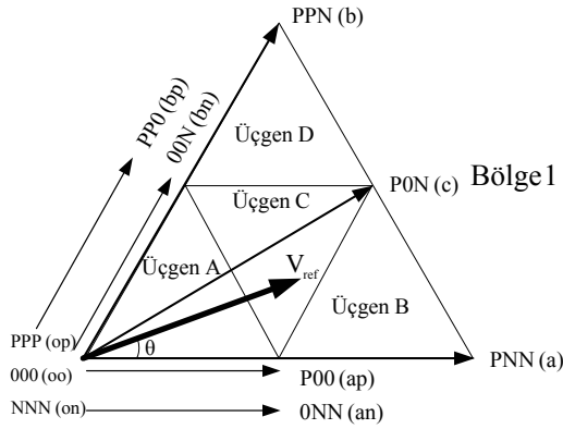
Şekil 3 Üç-düzeyle evirici çıkış gerilimi uzay vektör gösterimi (altgende ilk 60°).
