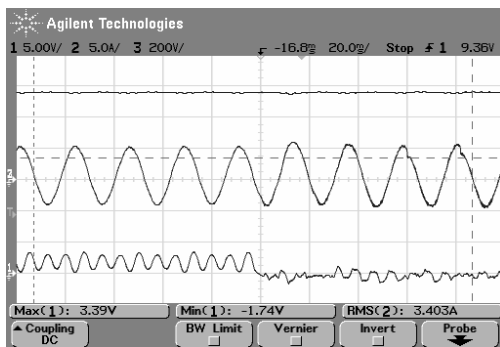
Şekil 12 M_i=0.87 çalışma noktasında DC bara toplam gerilimi, motor faz akımı ve nötr nokta gerilimi (Ölçekler: 5V/bölme, 5A/bölme, 200V/bölme, 20ms/bölme).
