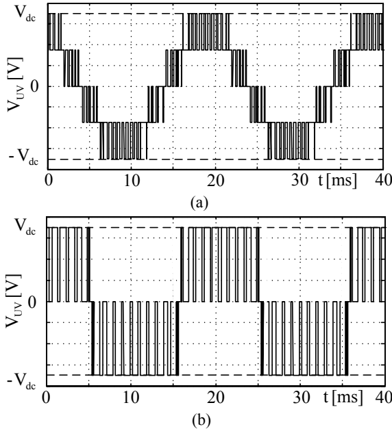
Şekil 2 Faz arası çıkış gerilimleri; (a) üç-düzeyle evirici, (b) iki-düzeyle evirici.
