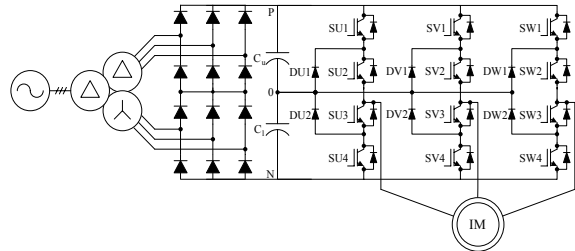
Şekil 13 Üç-düzeyleyici motor sürücü diyagramı.
