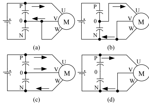
Şekil 6 Üç-düzeyle evirici anahtarlama durumlarının nötr noktası gerilimine etkilerini gösteren örnek durumlar.
